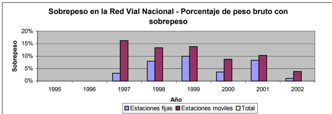
Figura 3. Graficas de la variación de los sobrepesos en Colombia. (Fuente – Subdirección de Conservación del INVIAS)
