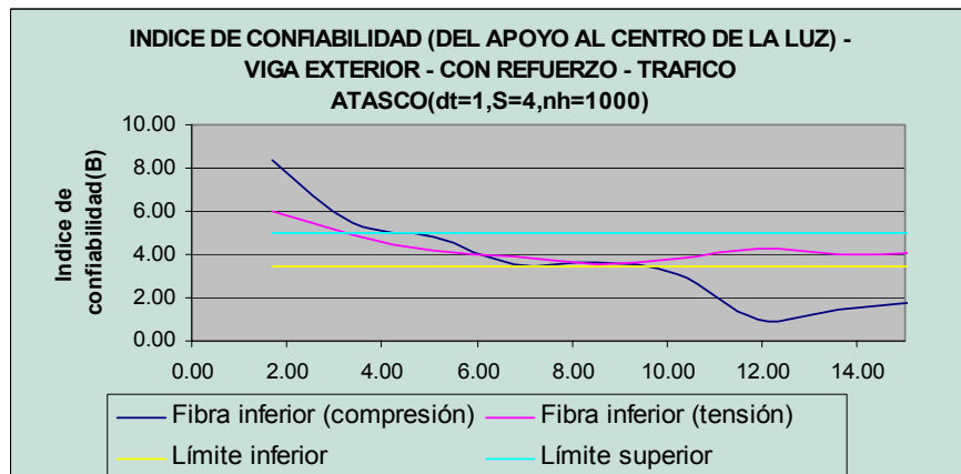
Figura 8. Variación de la confiabilidad para puente original con refuerzo
