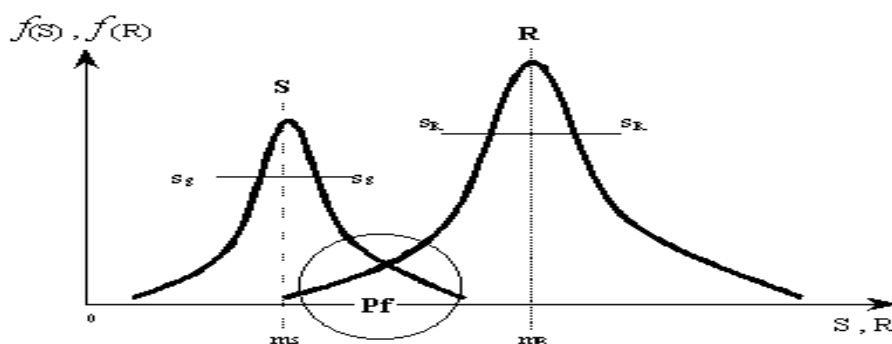
Figura 2. Curva de confiabilidad.
