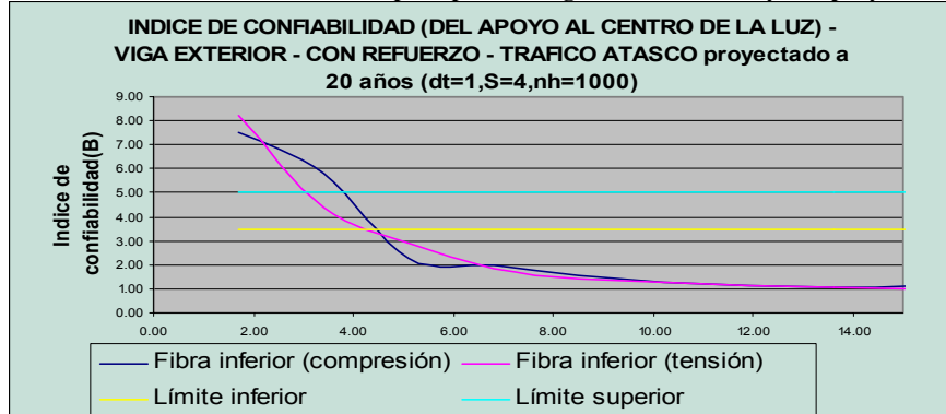
Figura 9. Variación de la confiabilidad para puente original con refuerzo y con proyección
