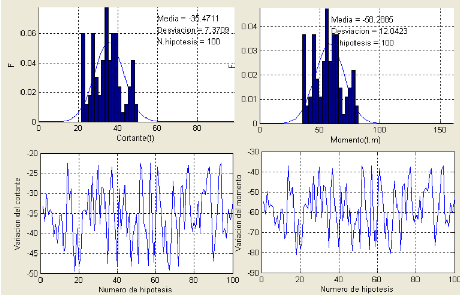
Figura 6. Caso de atasco, 100 hipótesis para una proyección de la carga de tráfico de 20 Años.
